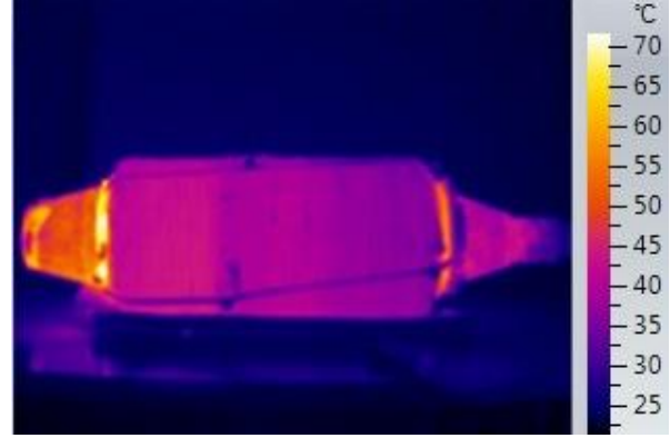
Şekil 3.1 İndüksiyonlu Akışkan Isıtıcısı Kovan Kısımının Sürekli Rejime Girdiği Andaki Termal Kamera Görüntüsü
