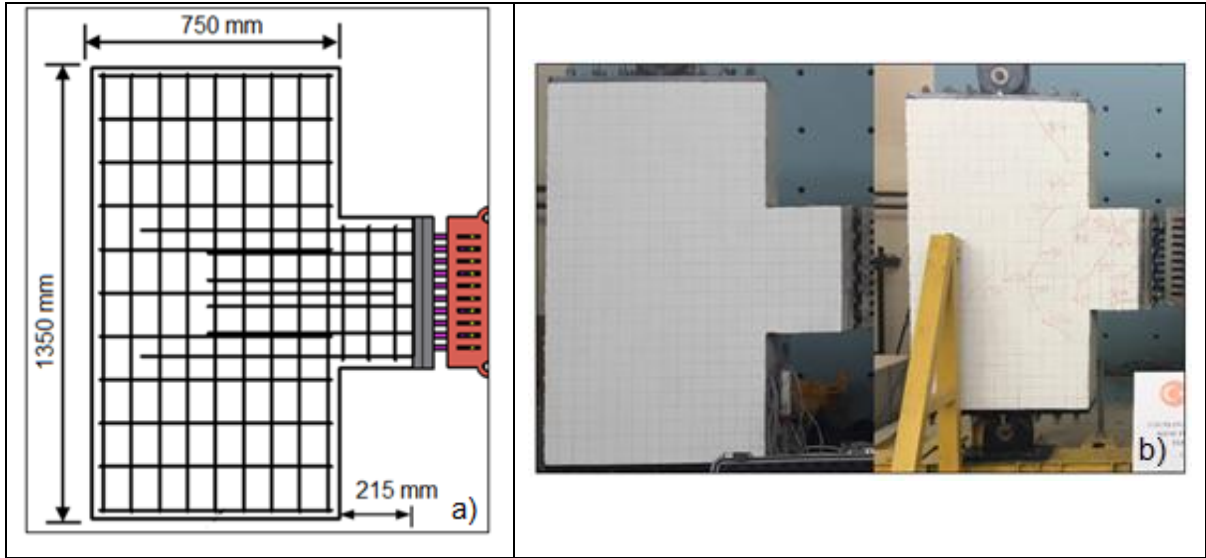
Şekil 3. a) Jeofizik ölçüler alınan betonarme yapı elemanının şematik görünümü b) Ölçüm yapılan betonarme yapının deneyden önceki ve sonraki durumu. Ölçüm hatları ve uygulanan yük sonrası oluşan deformasyonlar yapılar üzerinde çizilmiştir.
