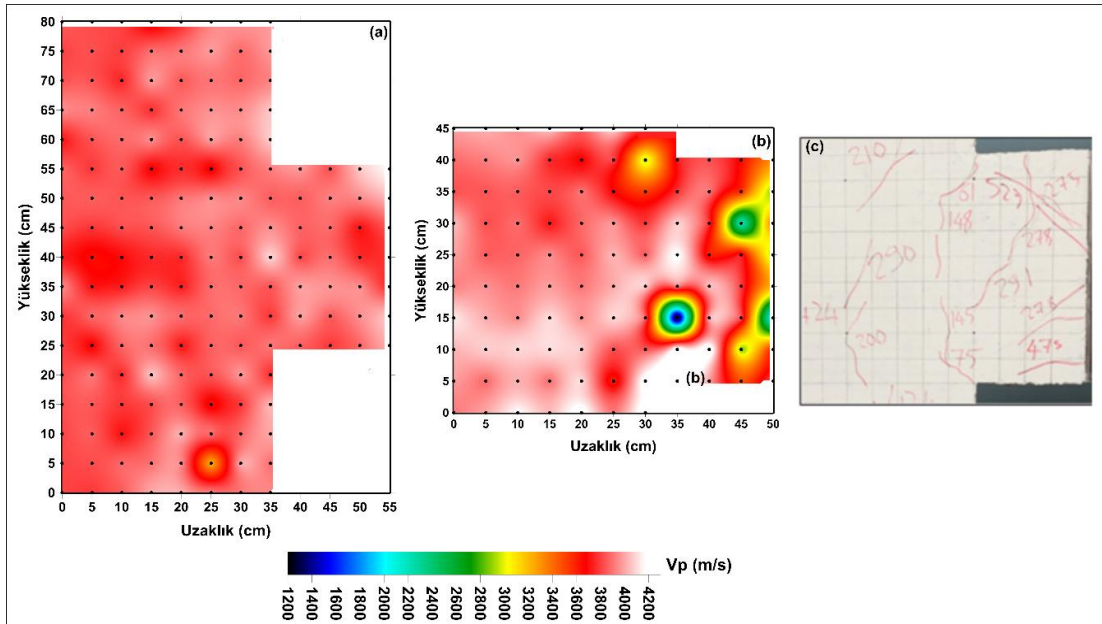
Şekil 4. Betonarme yapı üzerinde elde edilen ultrasonik boyuna dalga hız haritaları. (a) kuvvet uygulamadan önce, (b) kuvvet uygulandıktan sonra, (c) Betonarme yapıya gerilme uygulandıktan sonra deformasyonların gözlemlendiği kısım. Deformasyon sonrası ölçüler bu kısımda alınmıştır.
