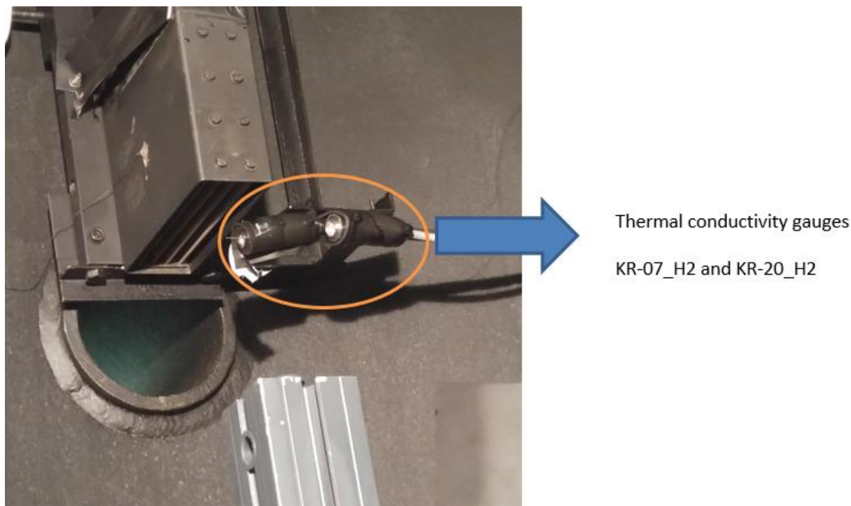
Figure 5 Hydrogen sensors at PAR inlet
